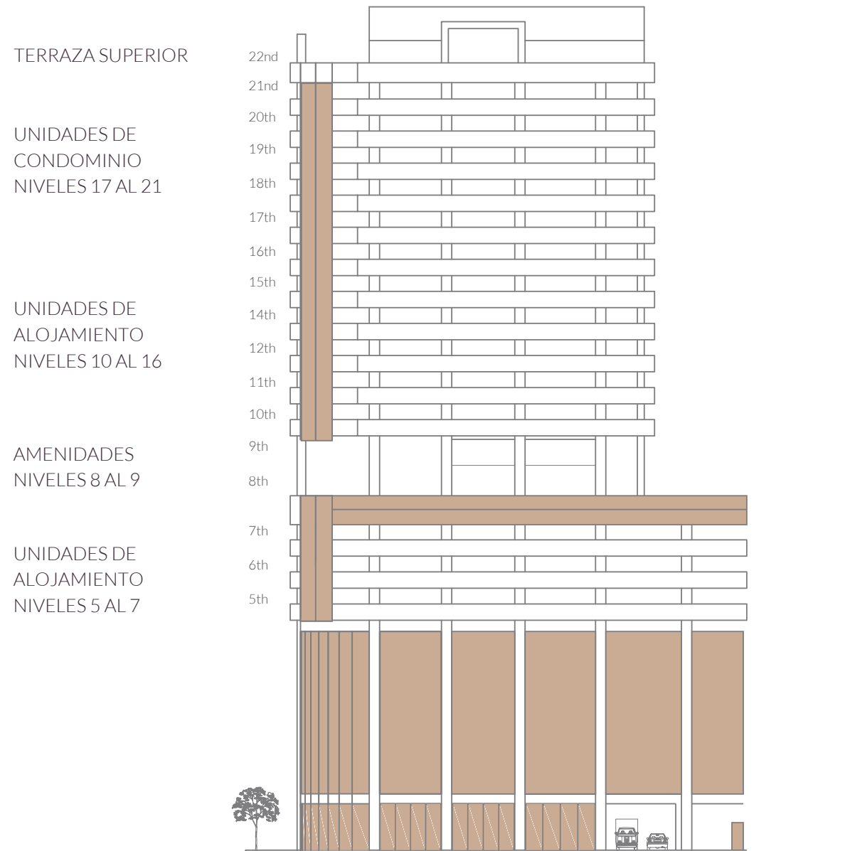
ALZADO NORTE
