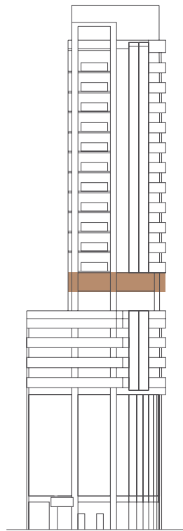
ALZADO ESTE
