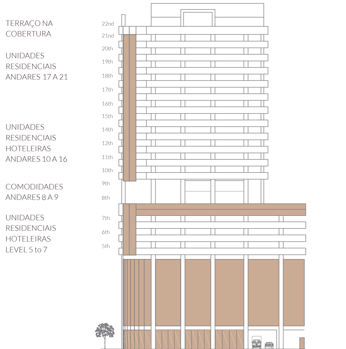
ELEVAÇÃO NORTE
